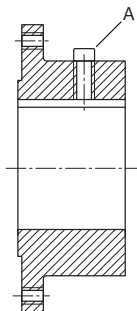
15 ábra: A állítócsavar az axiális rögzítéshez
