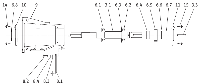
28 ábra: Csapágytartó
