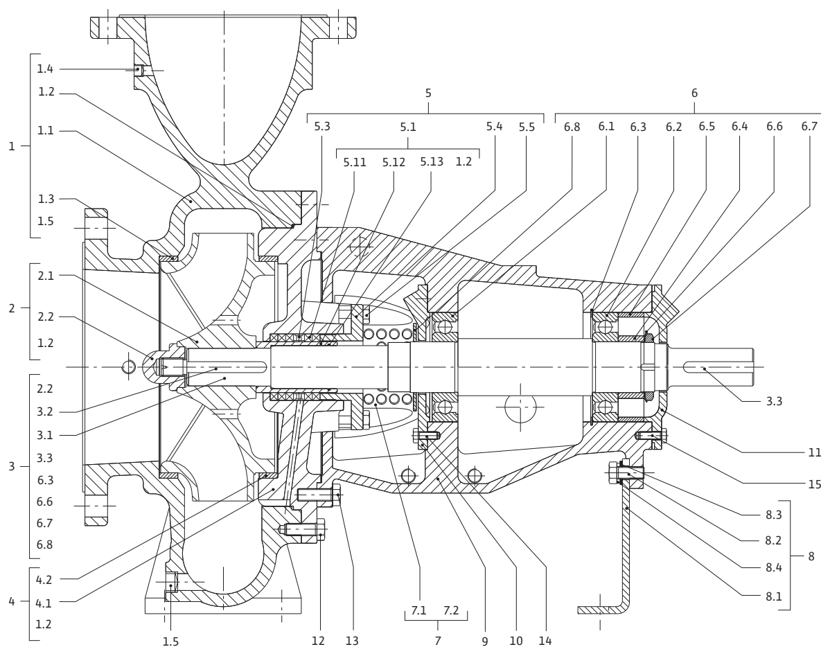
38 ábra: Wilo-CronoNorm-NLG tömszelencés tömítéssel
