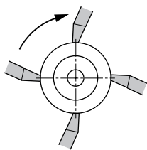
14 ábra: Az axiális beállítás ellenőrzése tolómérővel – a teljes kerületen
