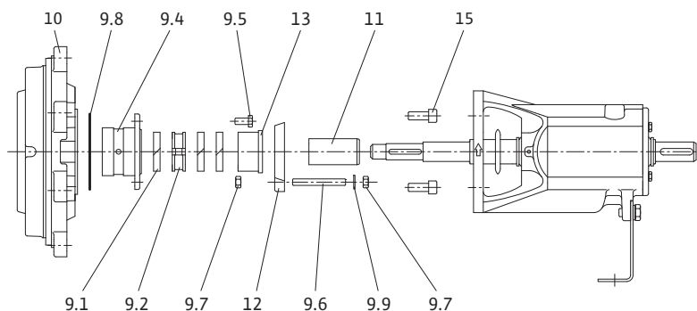
21 ábra: Tömszelencés tömítéses kivitel
