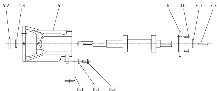
22 ábra: Csapágytartó
